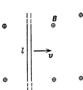
Рис. 19.1. Проводник длиной l движется с постоянной скоростью v перпендикулярно линиям индукции B
