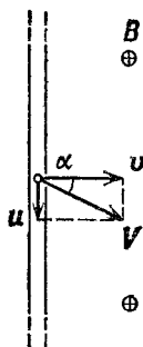
Рис. 19.2. Скорость V движения зарядов относительно лабораторной системы отсчета
