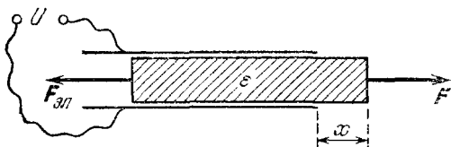
Рис. 11.1. К нахождению силы F_{\text{эл}} , втягивающей диэлектрическую пластину при неизменном напряжении U между обкладками конденсатора
