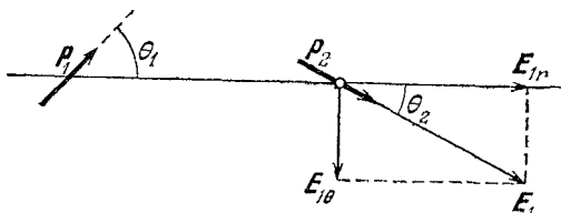
Рис. 6.1. Свободный диполь p_2 ориентируется вдоль напряженности поля E_1 , создаваемого закрепленным диполем p_1
