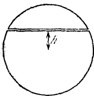
Рис. 8.1. Заряженный металлический шар разрезан на две части
