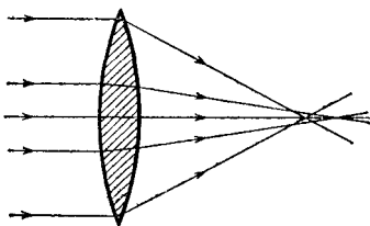
Рис. 6.1. Сферическая aberrация обыкновенной линзы
