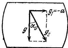
Рис. 10.2. В системе отсчета, связанной с цистерной, действует эффективное поле тяжести \mathbf{g}_2
