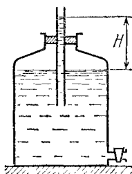
Рис. 5.2. При плотном закрывании пробки уровень воды в трубке поднимается
