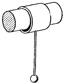
Рис. 4.1. Втулка маятника надета на неподвижную ось
